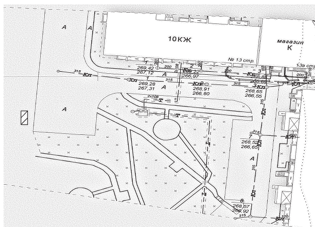
Схема размещения контейнерной площадки ул. Чкаловская, д.13
