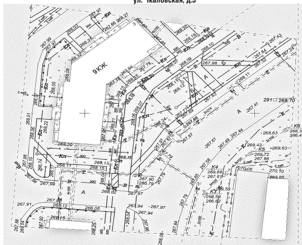
Схема размещения контейнерной площадки ул. Чкаловская, д.3
