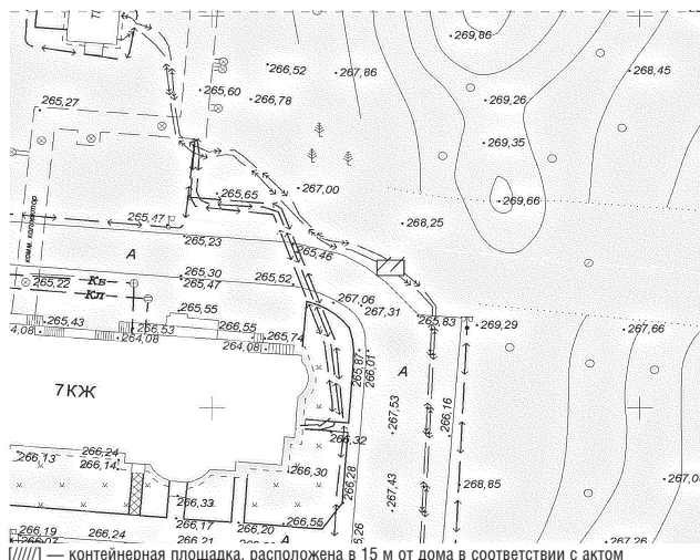
Схема размещения контейнерной площадки ул. Мира, д. 19
