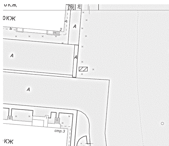
Схема размещения контейнерной площадки ул. Мира 19
